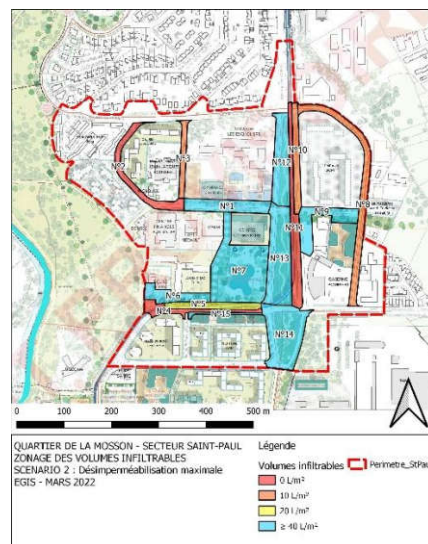
Exemple de répartition des volumes infiltrables sur le quartier Saint Paul Extrait présentation Quartier de la Mosson gestion des eaux pluviales 23/03/2022, Egis
