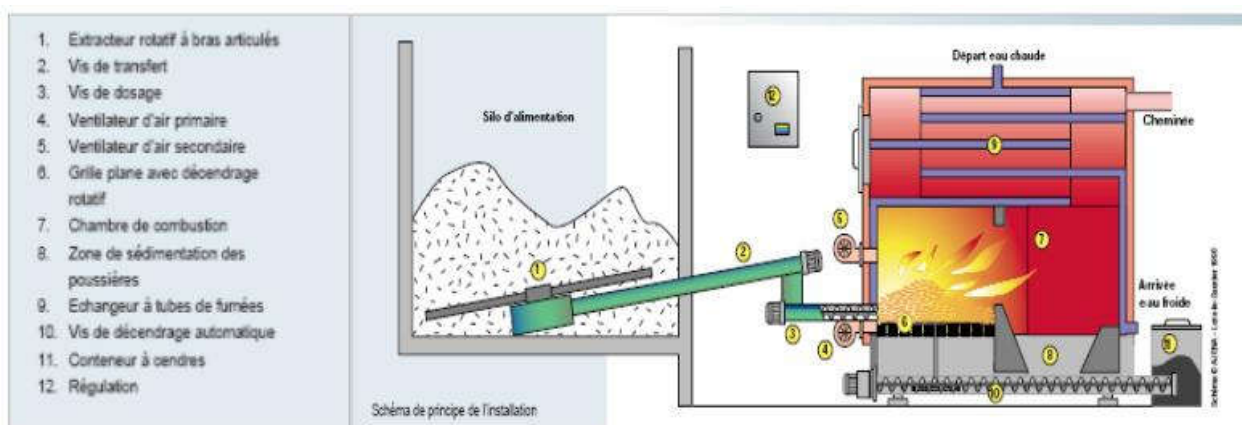
Schéma d'une chaudière bois
