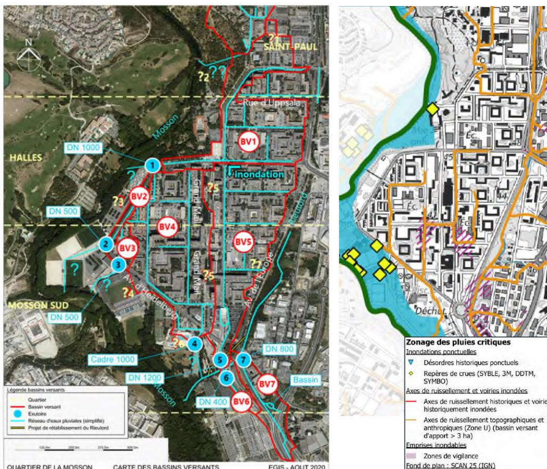
Extrait de la carte des bassins versants composant le réseau pluvial sur une large partie Sud du périmètre de la concession (gauche) ; identification des axes de ruissellement anthropiques et zones d'accumulation (droite)
