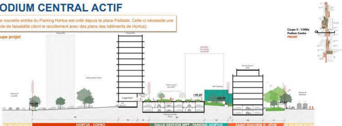
Coupe projet des espaces publics du podium central - Passagers des Villes
