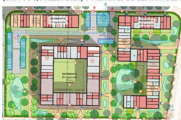
RÉSIDENCE SATURNE | VUE EN PLAN PROJET (GRPT PDV, JUILLET 2020) + PRINCIPES DE GESTION DES EP
