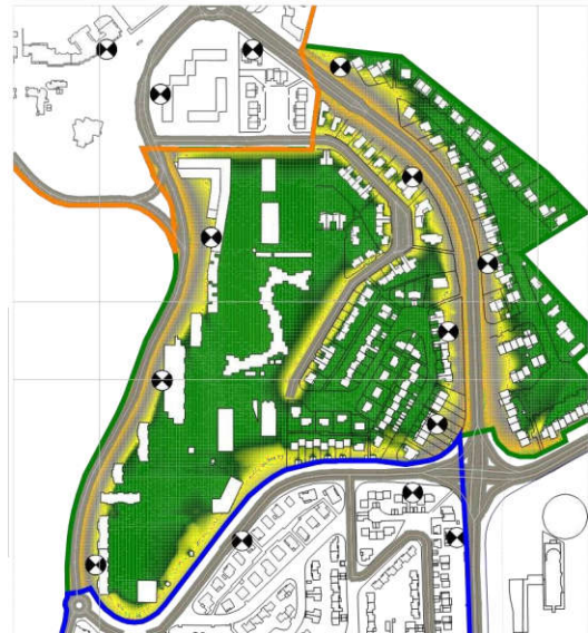
Cartes des isophones à 2m de hauteur pour la zone 3 à l'état initial, de jour et de nuit, Étude acoustique, Bet PIALOT-ESCANDE, Septembre 2022.
