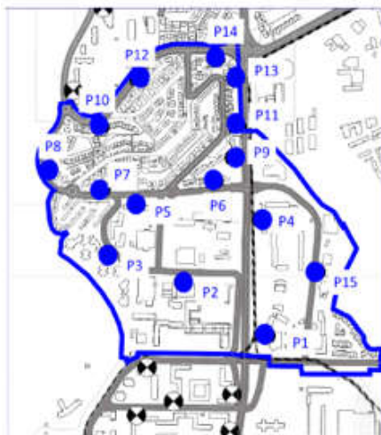
Synthèse des récepteurs placés en façades bâtiments de la zone 2, Étude acoustique, Bet PIALOT-ESCANDE, Juin 2022.
