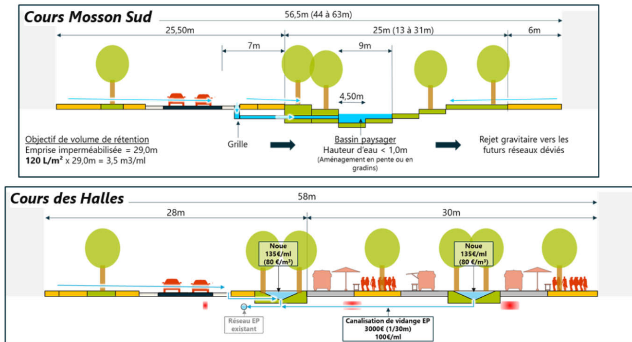
Coupes sur les secteurs d'espaces publics requalifiés Extraits Présentation Quartier de la Mosson gestion des eaux pluviales 23/03/2022, Egis
