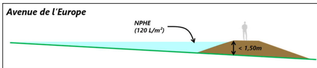
Coupe type des modalités de rétention pluviale envisageables sur l'Avenue de l'Europe Extrait Présentation Quartier de la Mosson gestion des eaux pluviales 23/03/2022, Egis
